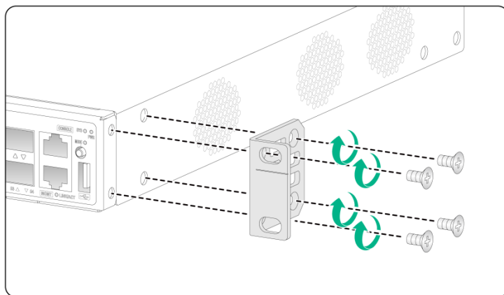
图2-9 安装挂耳到交换机示意图（端口侧，以 S5200-54S-EI-G 为例）
