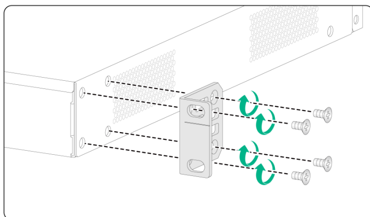
图2-10 安装挂耳到交换机示意图（电源侧，以 S5200-54S-EI-G 为例）
