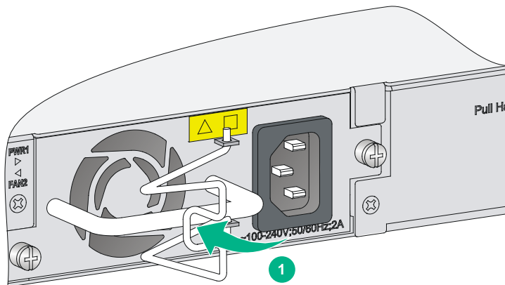
图2-22 LSPM2150A-Z 交流电源线连接示意图（一）
